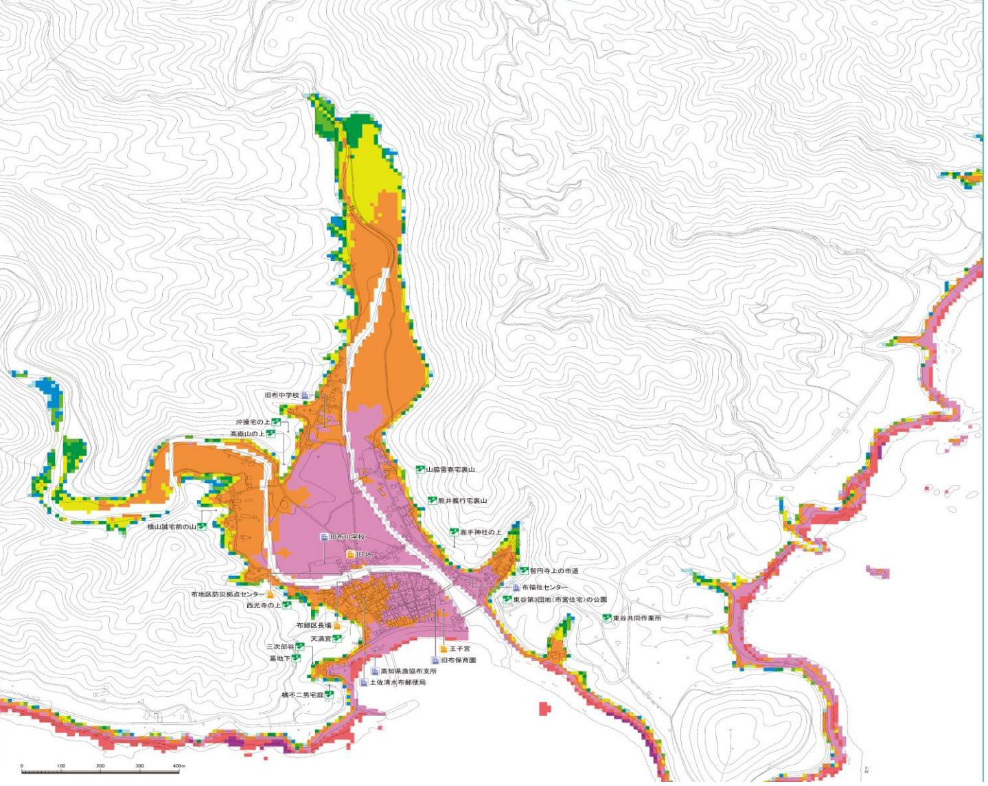
図 3.2 津波浸水予測図（東谷地区）
