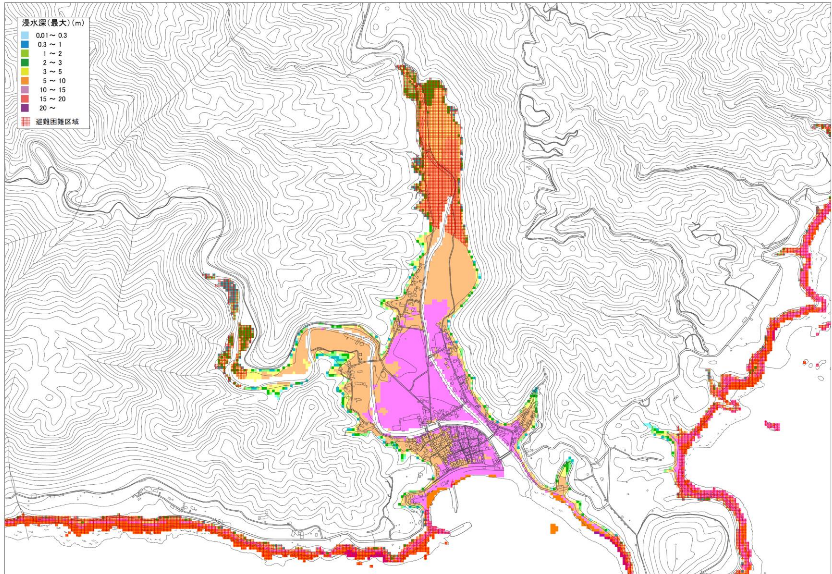
図 4.2 避難困難区域算定結果図(東谷地区)
